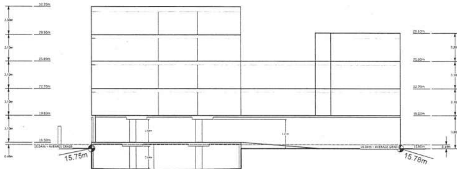
1 SECTION 1 A-13 Scale: 3/32" = 1'-0"
