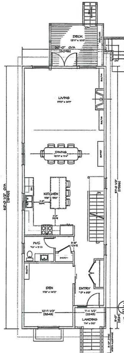
③ LOWER - New SFD Scale: 1/4" = 1'-0"
