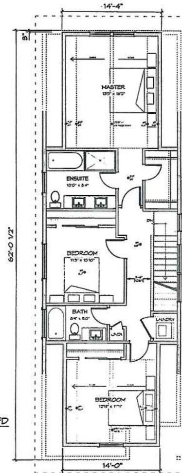
① UPPER - New SFD Scale: 1/4" = 1'-0"
